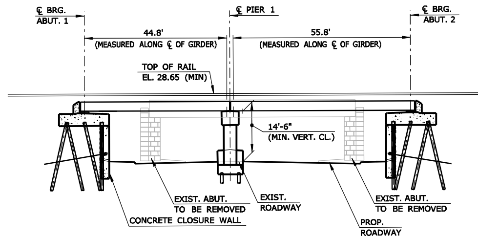
ELEVATION SCALE: 1" = 30'
