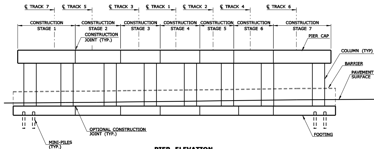
PIER ELEVATION SCALE: 1/16" = 1'-0"
