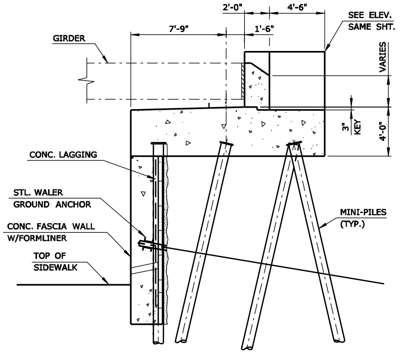
ABUTMENT SECTION SCALE: 1/8" = 1'-0"
