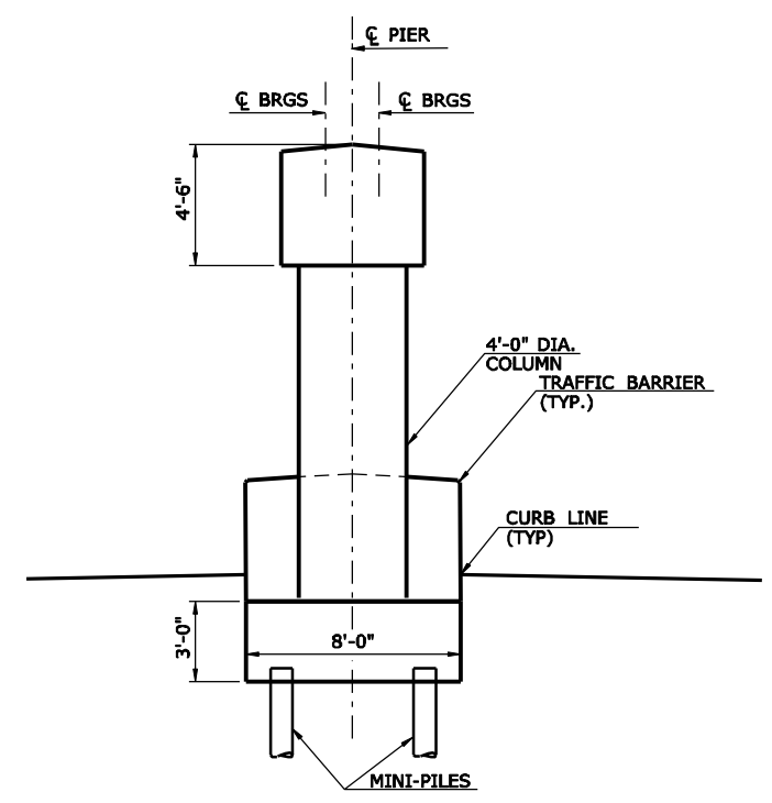
SECTION SCALE: 1/8" = 1'-0"
